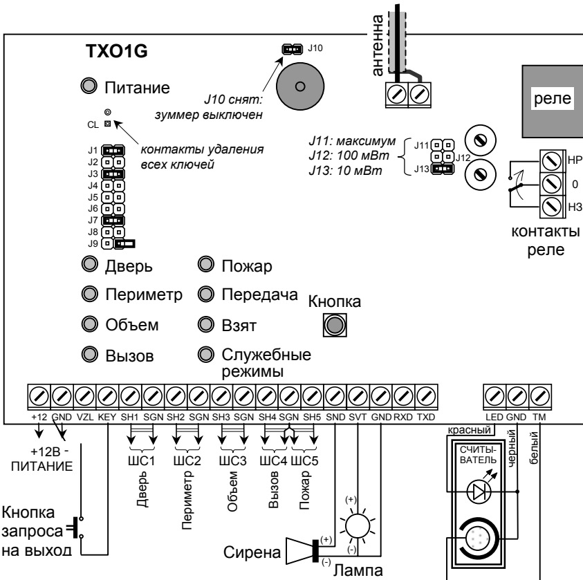
Рисунок 5. Монтажная схема передатчика
